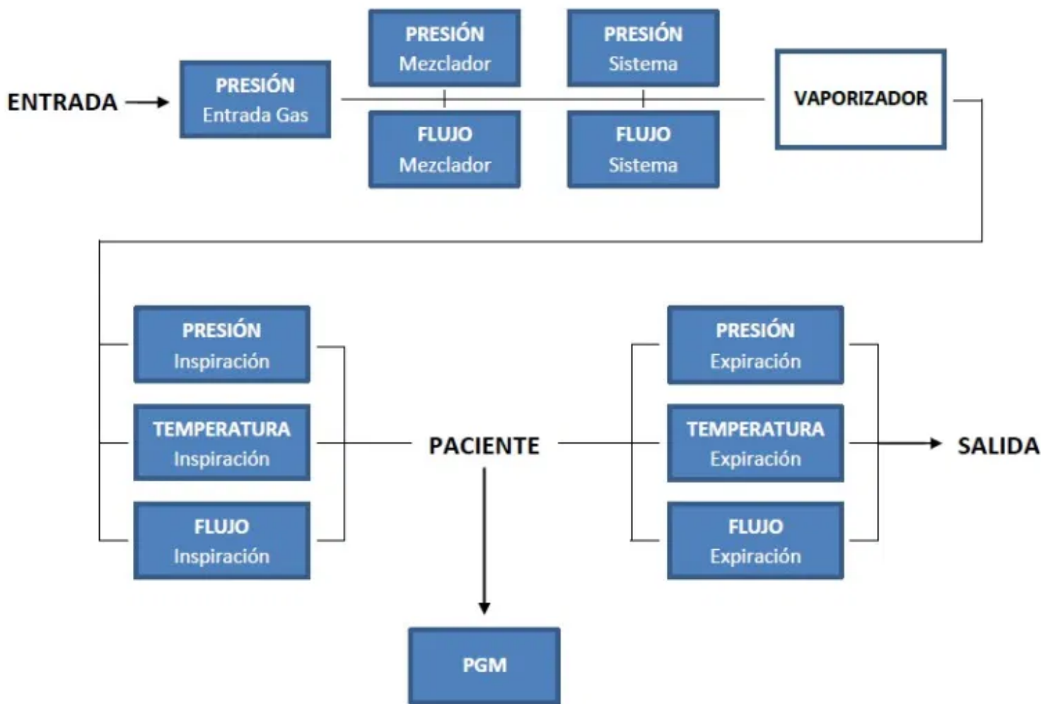
Figura 11: Esquema de flujo y sensores de DrägerPerseus A500..
